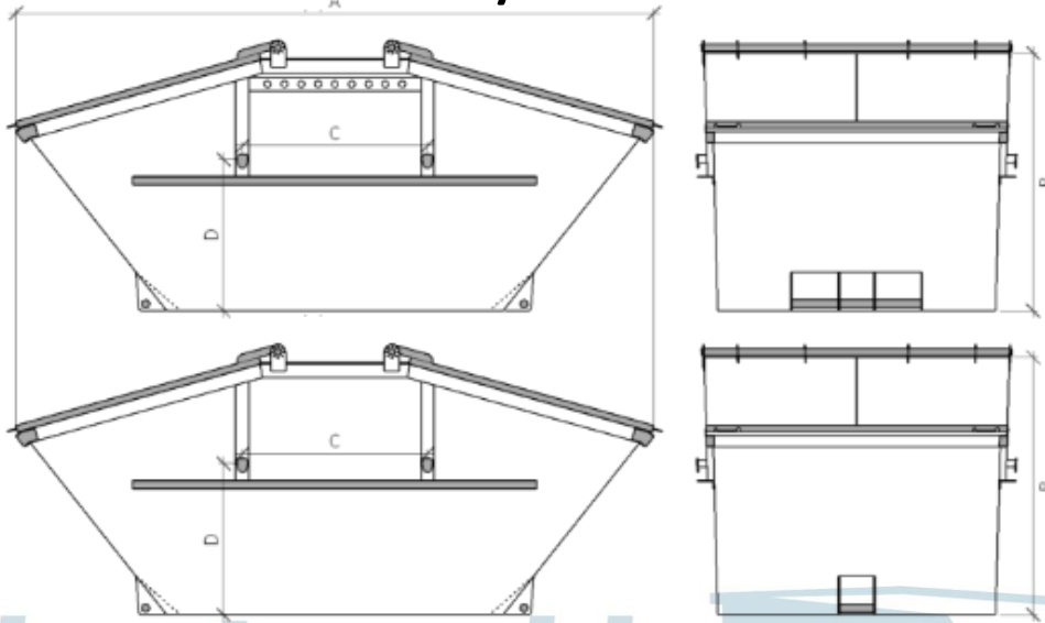
Abmessungen in Millimetern
